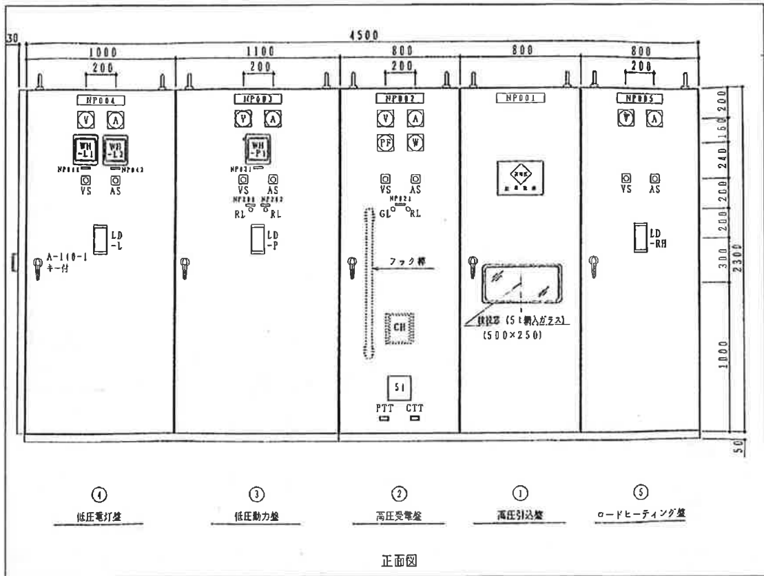
キュービクル正面図
