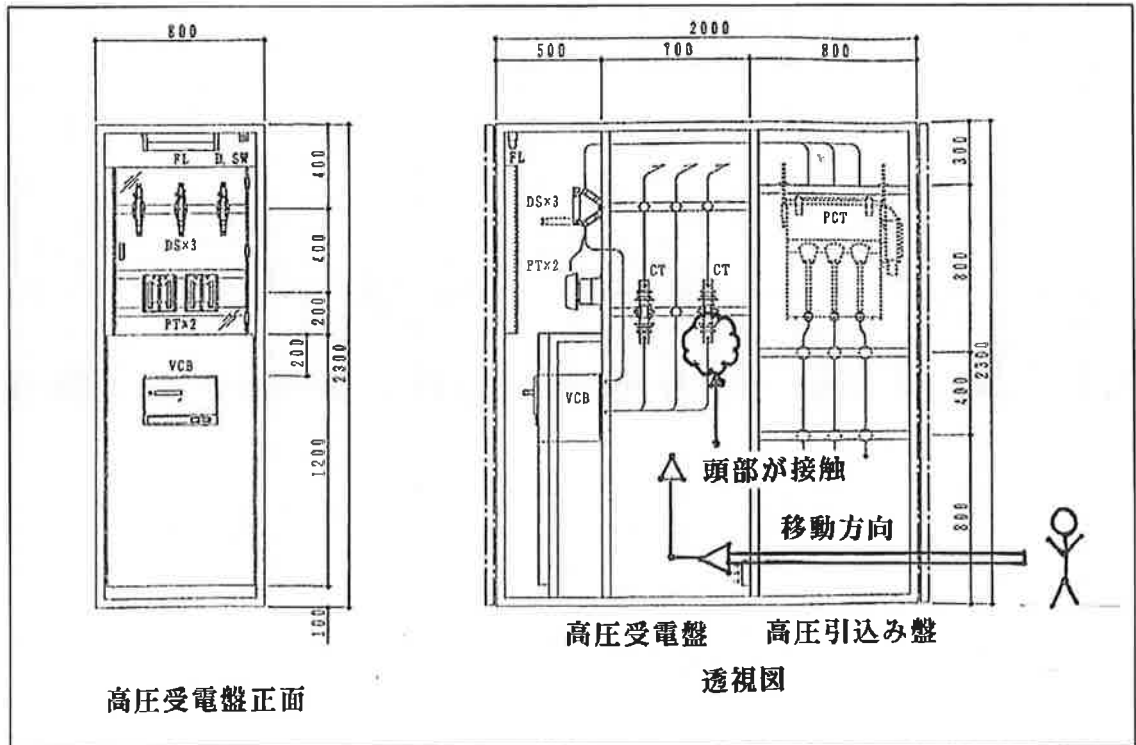
キュービクル正面図
